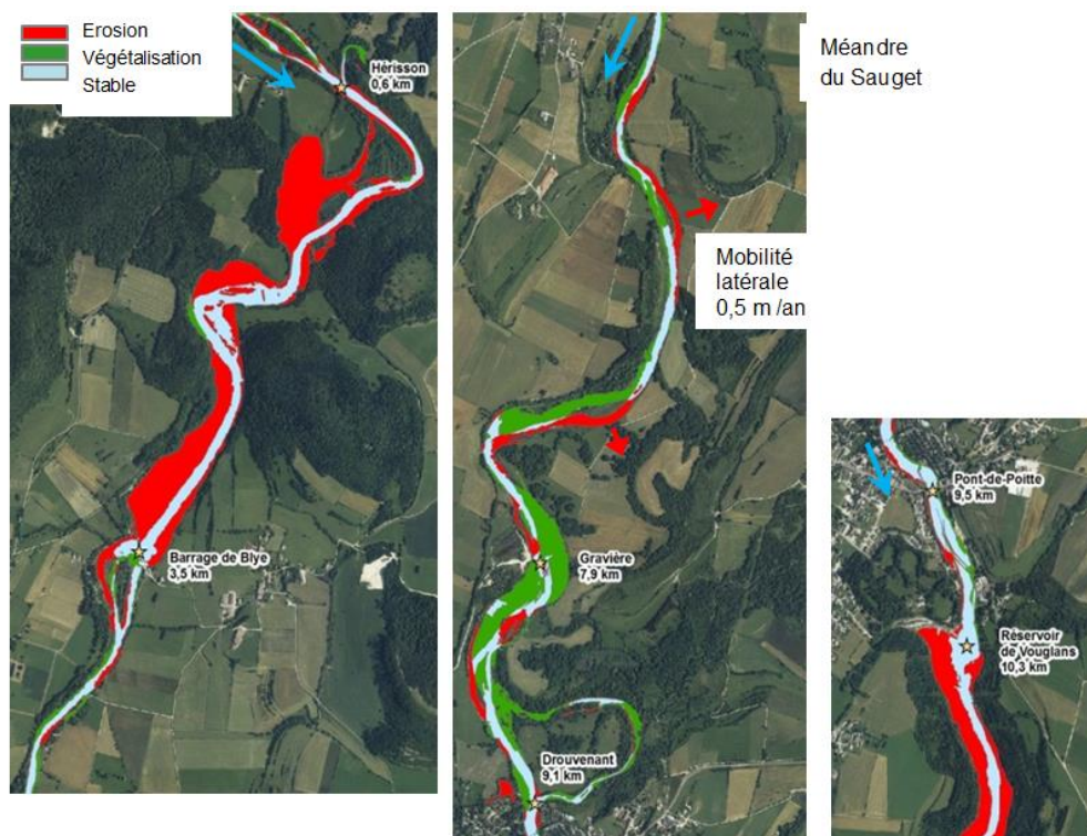
Figure 3 : Surfaces érodées, végétalisées et stables entre 1953 et 2010.
