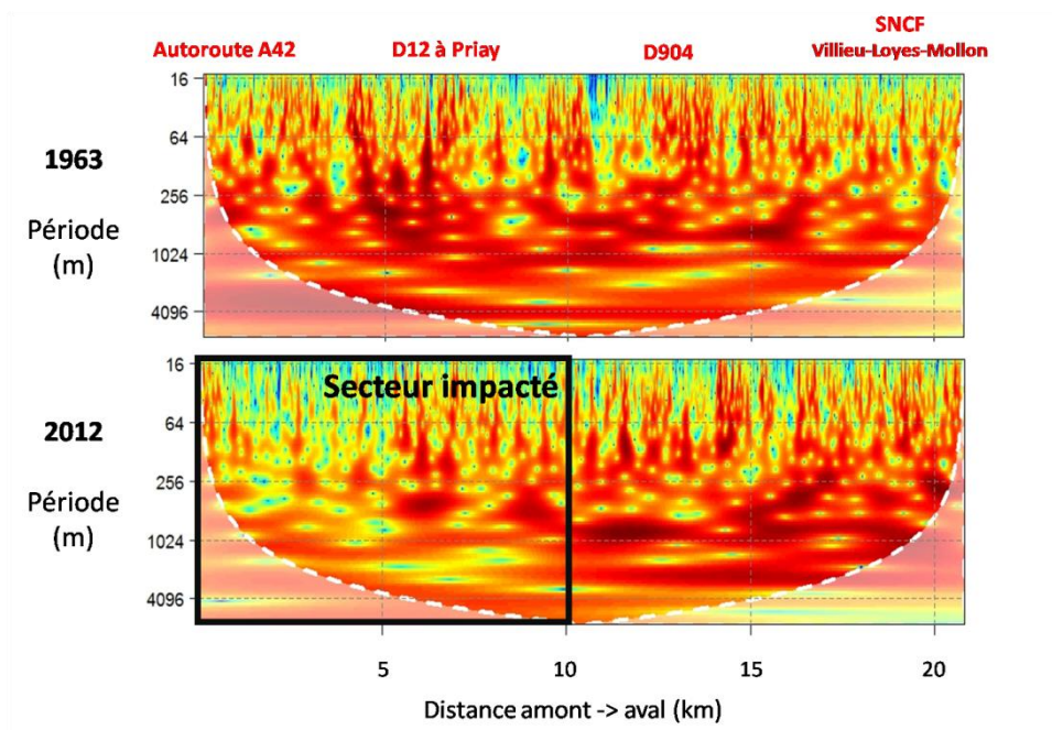
Figure 17 : Spectre de décomposition en ondelettes continues des signaux bathymétries de 1963 et 2012.
