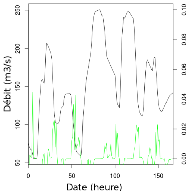
Figure 29 : Superposition de la chronique de débit horaire de la période 2-9 mars 2009 (noir ; échelle de gauche) et de la variabilité de la surface exondée (station-MdG) au pas de temps horaire (exprimée en % de la surface mouillée à chaque pas de temps ; vert ; échelle de droite) estimée à partir d'une simulation pseudo-stationnaire.
