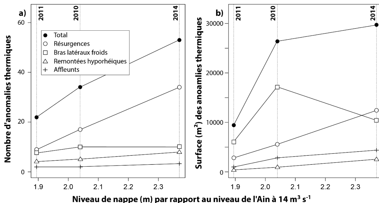
Figure 33 : Relations entre le nombre (a) et la surface (b) des anomalies thermiques et le niveau de nappe. Le niveau de nappe correspond au niveau moyen à Saint-Maurice-de-Rémens et Chazey-sur-Ain par rapport au niveau de la rivière à 14 m³ s⁻¹. Voir la Figure 2.1 pour l'emplacement des stations. Les données d'altitude de la rivière proviennent de Naudet et al. (2014).
