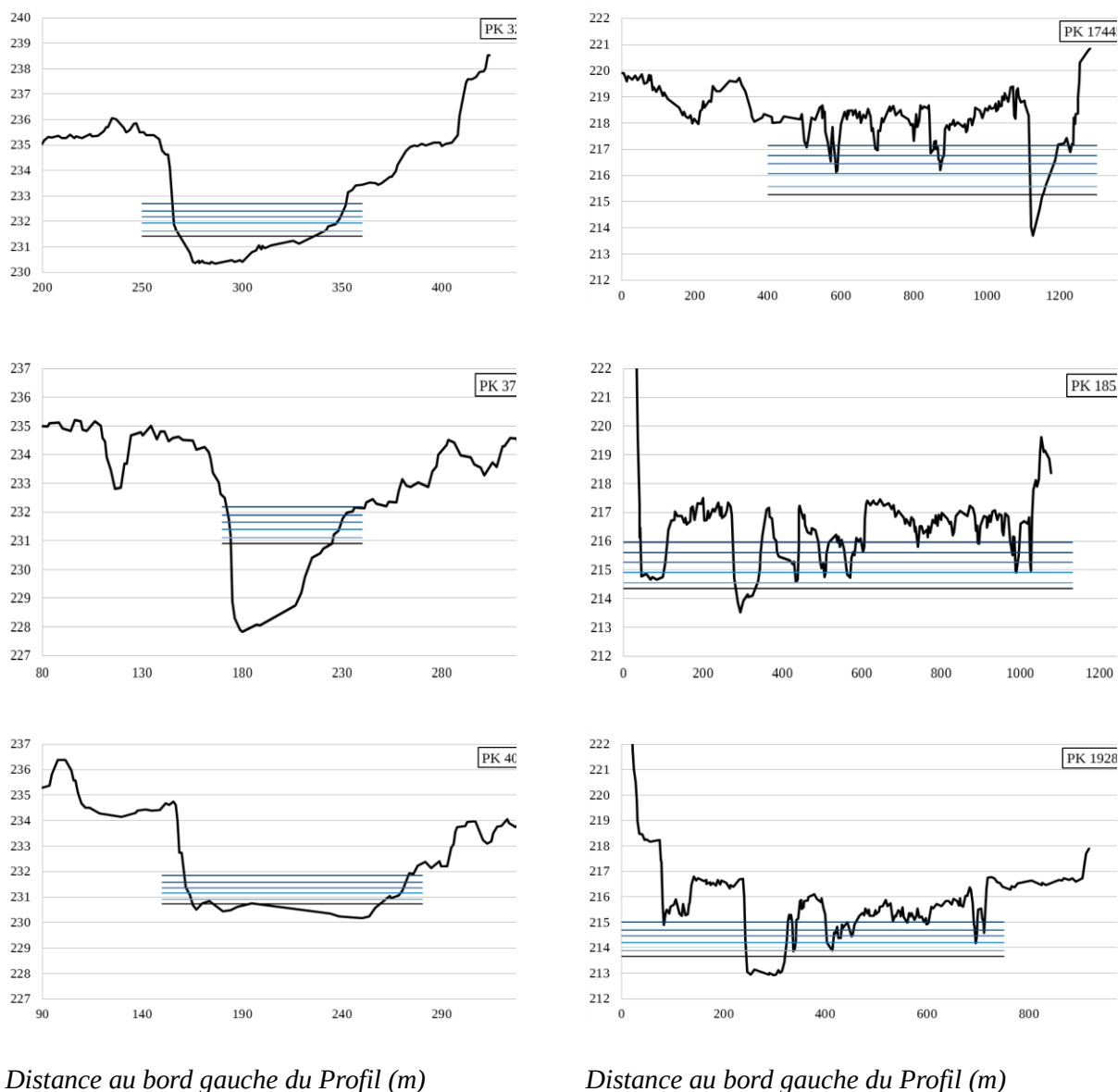
Figure 22 : Evolution du niveau d'eau (Altitude en m) sur trois des cinq profils en travers pour 20, 40, 80, 125, 175 et 250 \text{m}^3.\text{s}^{-1} (niveau d'eau évoluant de bas en haut) de chaque station (amont à gauche et aval à droite).
