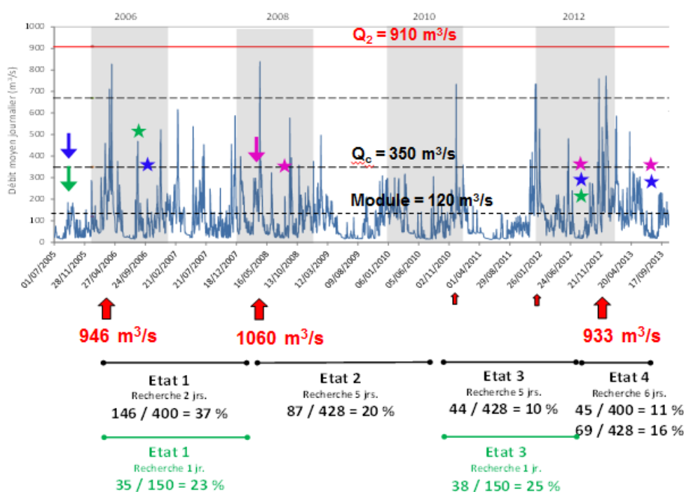
Figure 8 : Chronologie du suivi RFID de Gévrieux et Varambon (2005-2013) : dates de déploiement (flèches) et de recherche (étoiles) des PIT tags (station hydrométrique de Chazey-sur-Ain).
