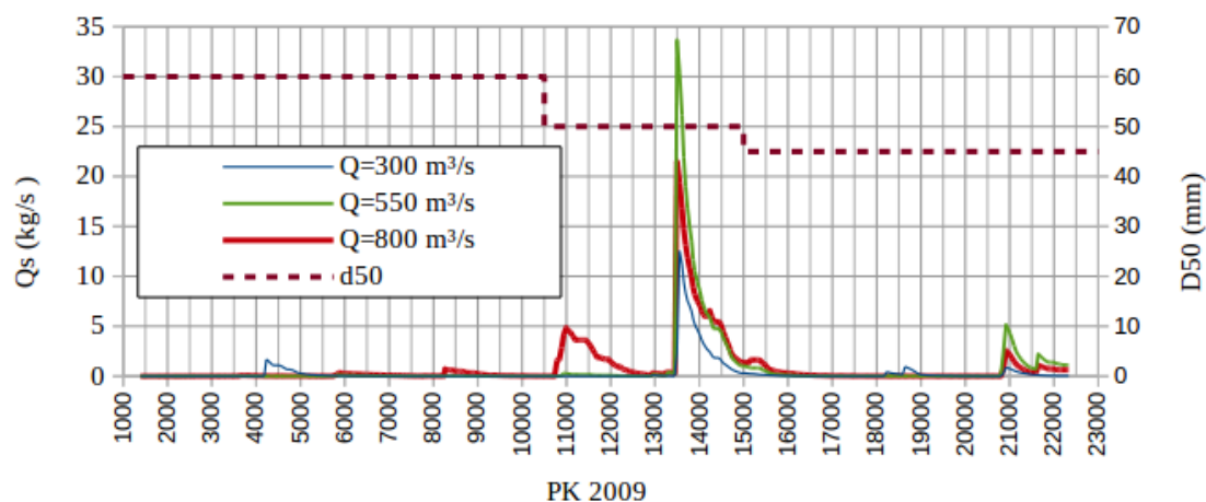
Figure 13 : Profil en long du transport solide modélisé avec le modèle 1D pour une granulométrie grossière.
